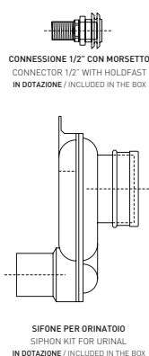
SIFONE PER ORINATOIO SIPHON KIT FOR URINAL IN DOTAZIONE / INCLUDED IN THE BOX
