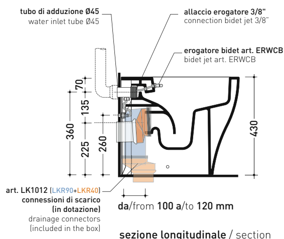
sezione longitudinale / section
