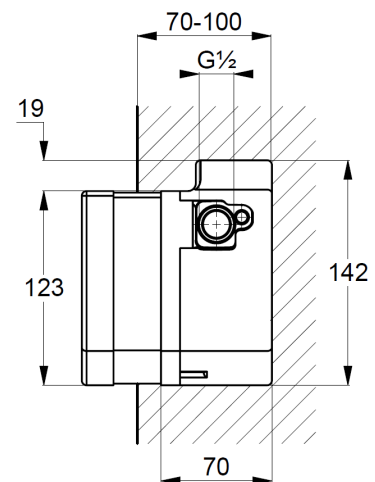
РАЗМЕРЫ
