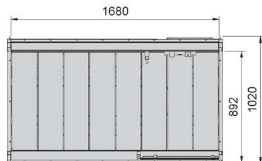
SEZ. A-A
