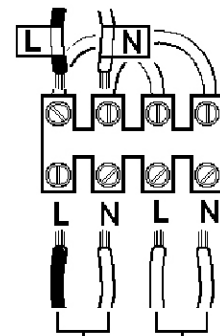
التسليك من خلال مصدر التيار CABLAGGIO PASSANTE ALIMENTAZIONE POWER SUPPLY FEEDTHROUGH WIRING CABLEADO PASANTE CEBADOR
